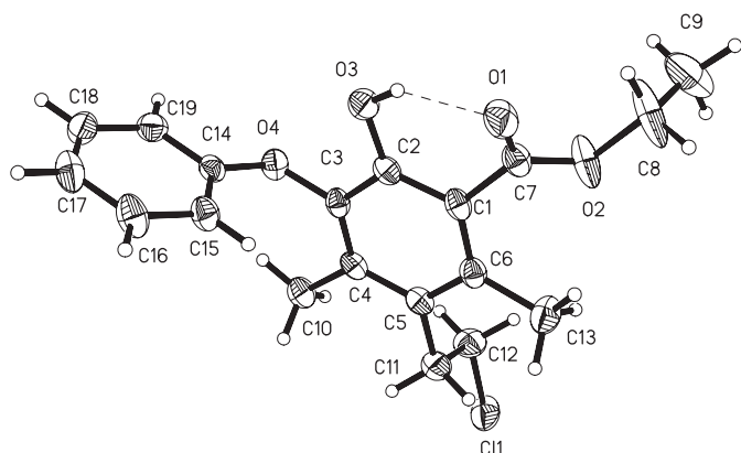
Figure 2. Ortep plot of 9a .
